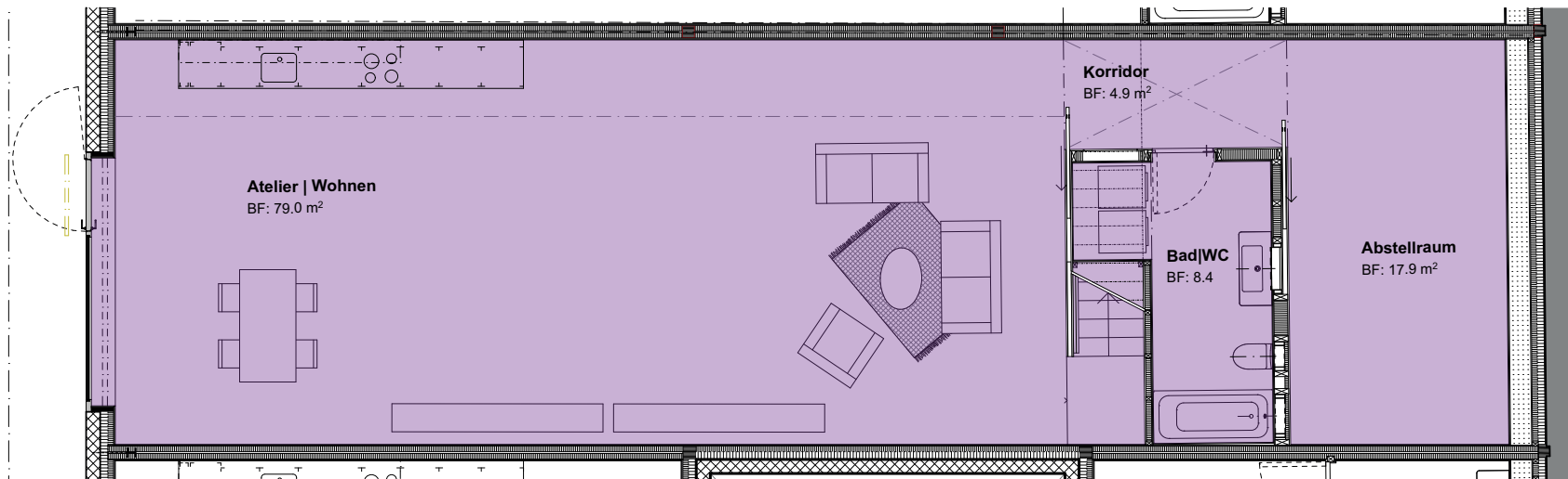
Erdgeschoss
